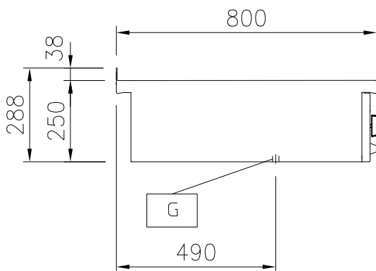
Zij aanzicht
