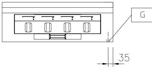
Front aanzicht
