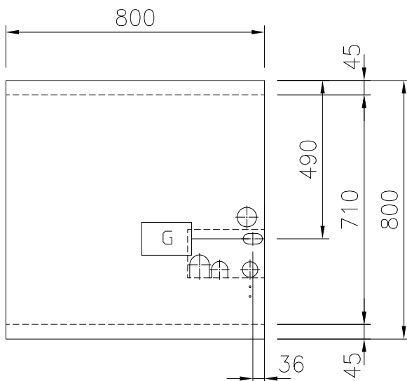
Boven aanzicht
